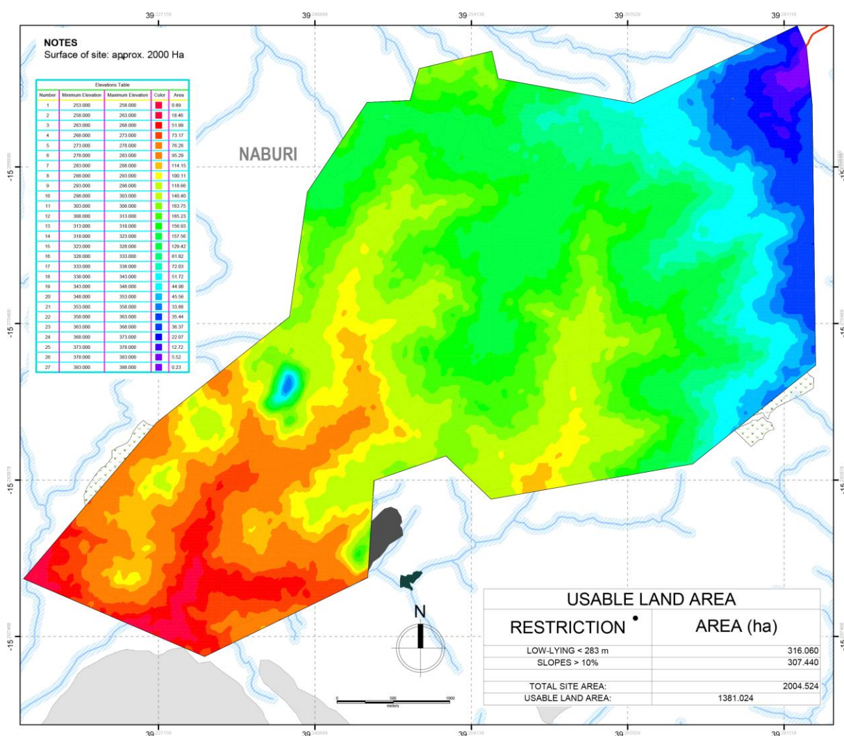
Mapa 7 Análise da topografia do Centro de Marratane Fonte: Adaptado de UNHCR (2017)
