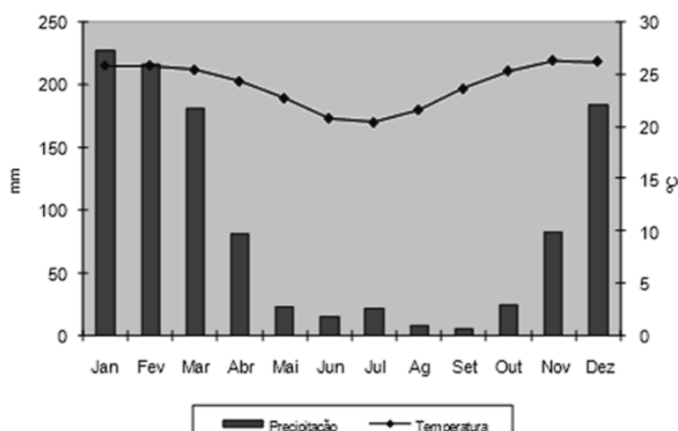
Gráfico 8: Pluviosidade e temperatura médias mensais da Província de Nampula; Fonte: TRINDADE (2013)
