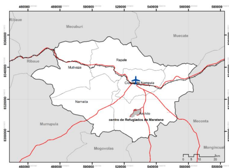
Mapa 3 Localização do centro de refugiado de Maratane Fonte: Autores
