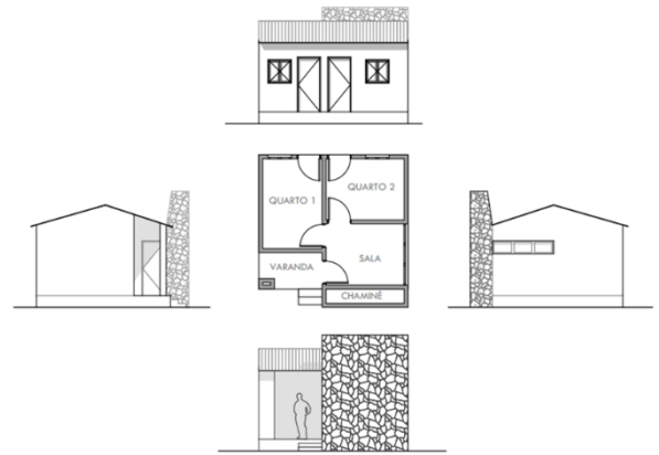
Figura 10 Tipologia das habitações contruídas com técnicas de construção convencional Fonte: Autores (2017)
